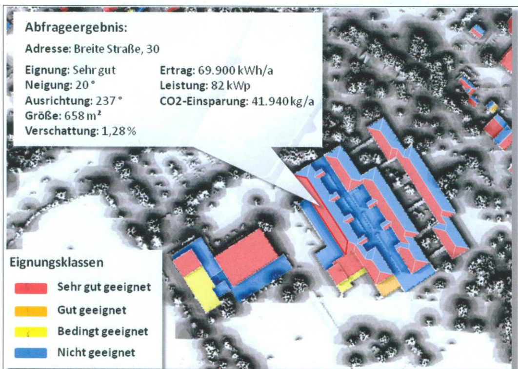
Die Abbildung zeigt an einem Beispielgebäude wie das fertige Solardachkataster in Bernkastel-Wittlich aussieht. Über eine Legende unten links im Bild ist die Eignung der einzelnen Dachseiten für Photovoltaik leicht abzulesen
